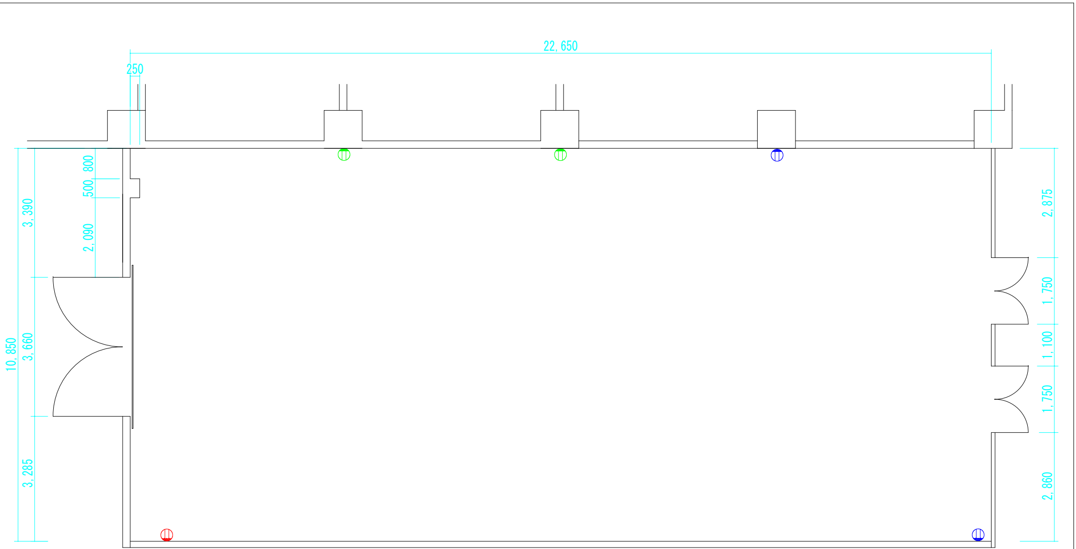
小ホール (CH=3600)
