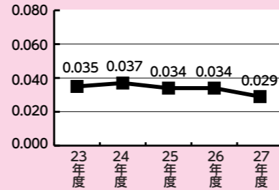
■二酸化窒素濃度経年変化（年平均値）（単位：ppm）
