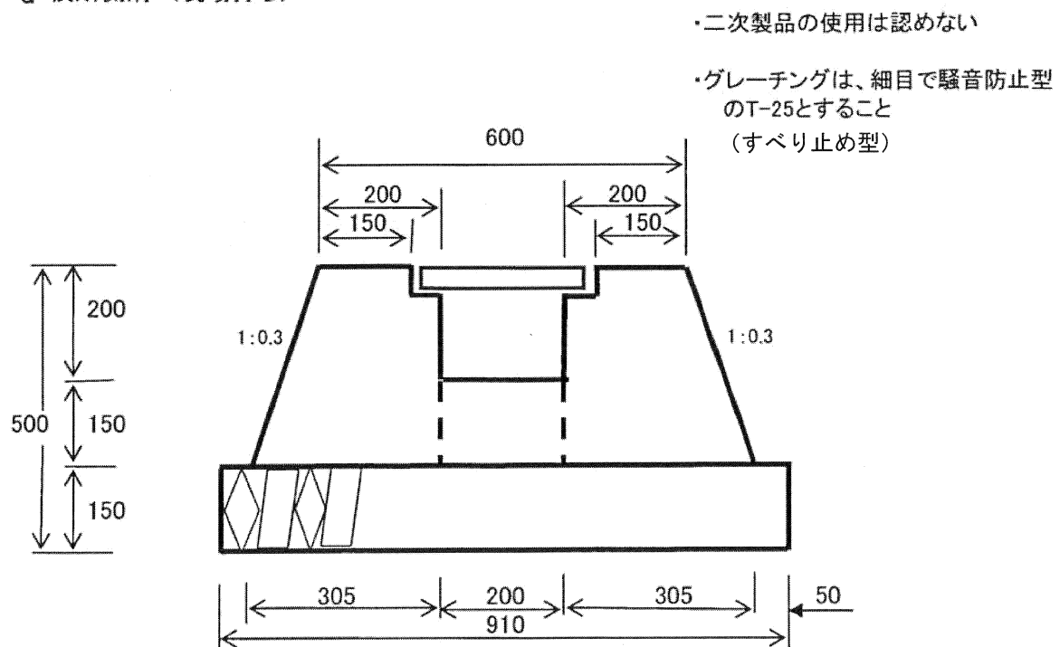
d 横断側溝（現場打ち）
