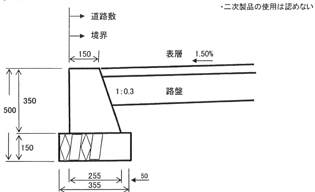
c 舗装止め（現場打ち）
