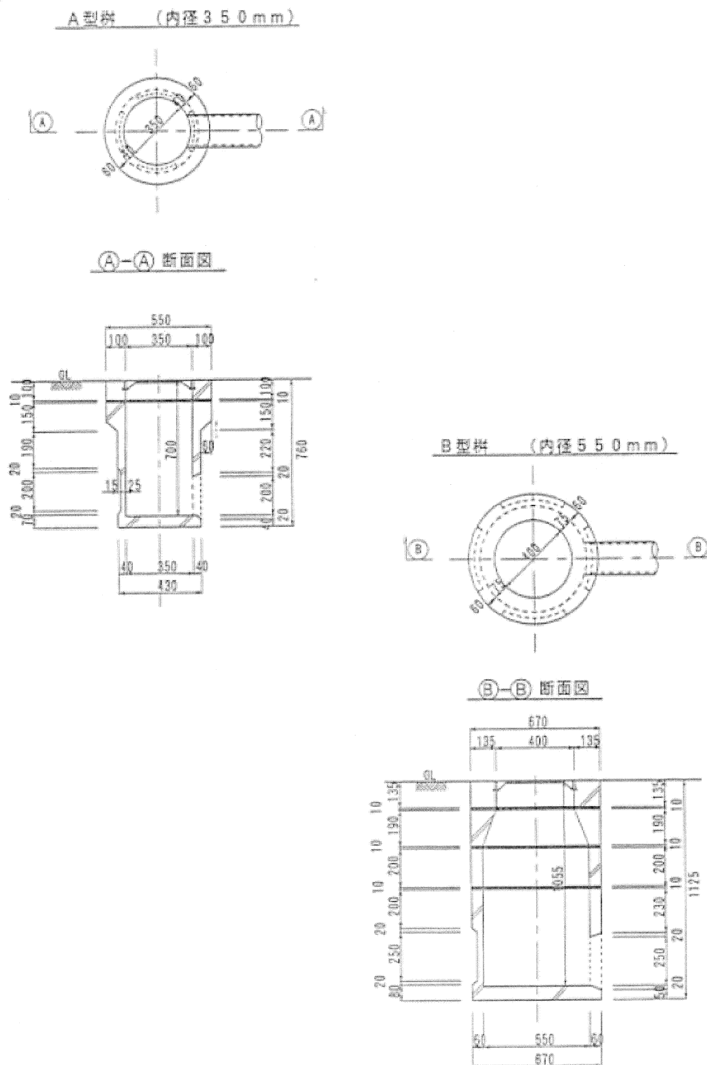
別図 1 0 汚水枡標準構造図 (A型枡・B型枡)
