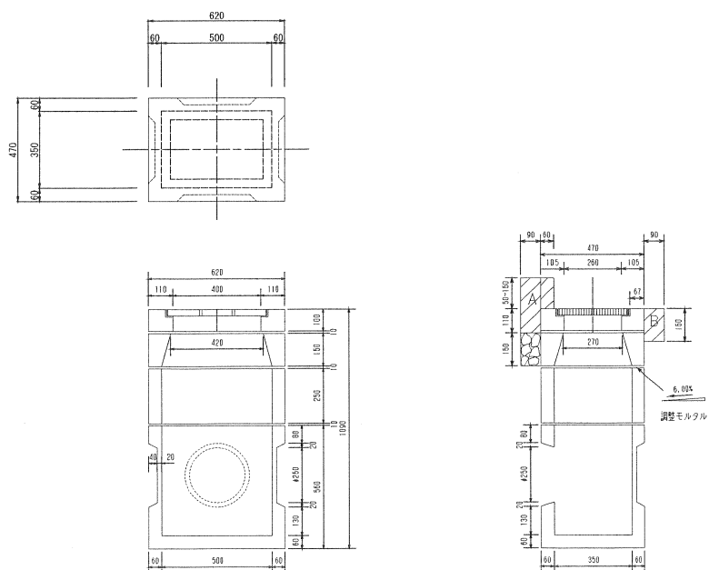
雨水L型枳標準構造図
