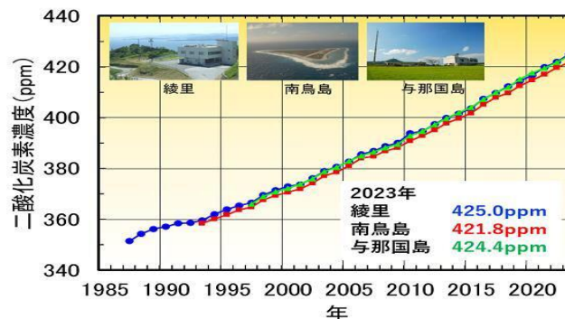
【二酸化炭素濃度の変化】
