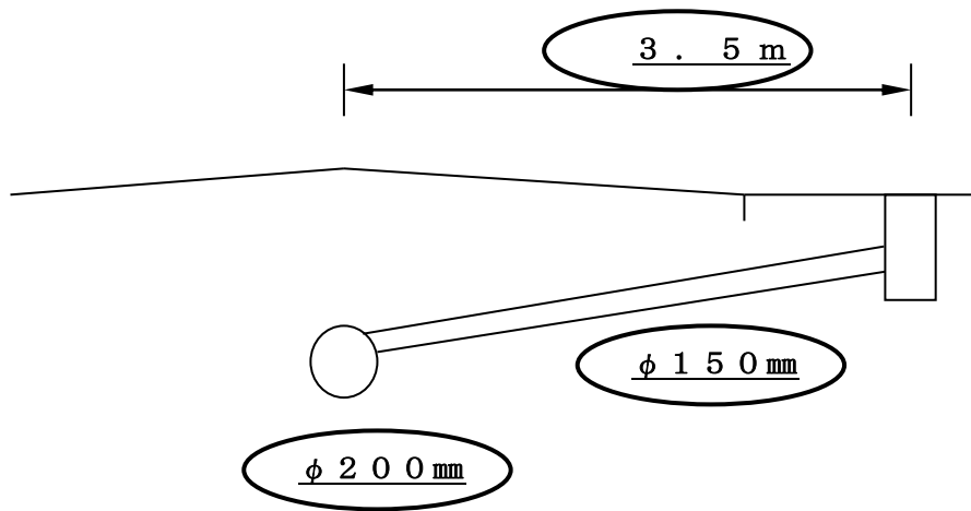
断面図
